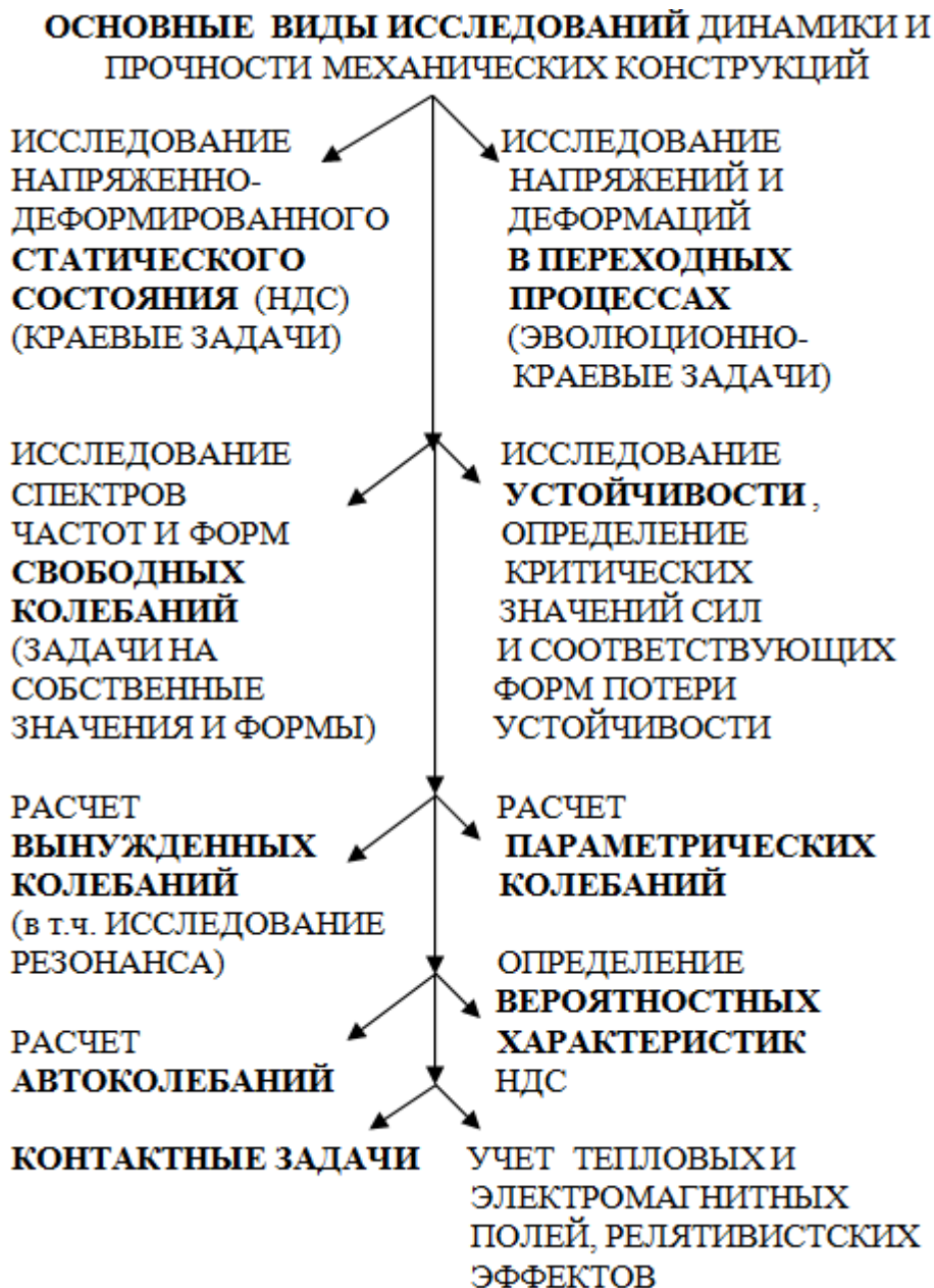
Рисунок 4 – Основные виды исследований моделей АТ и СТО
