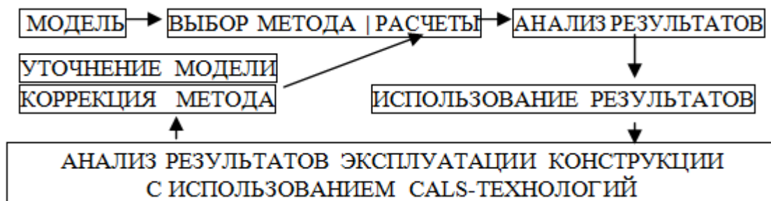
Рисунок 1 – Общая схема математического моделирования
