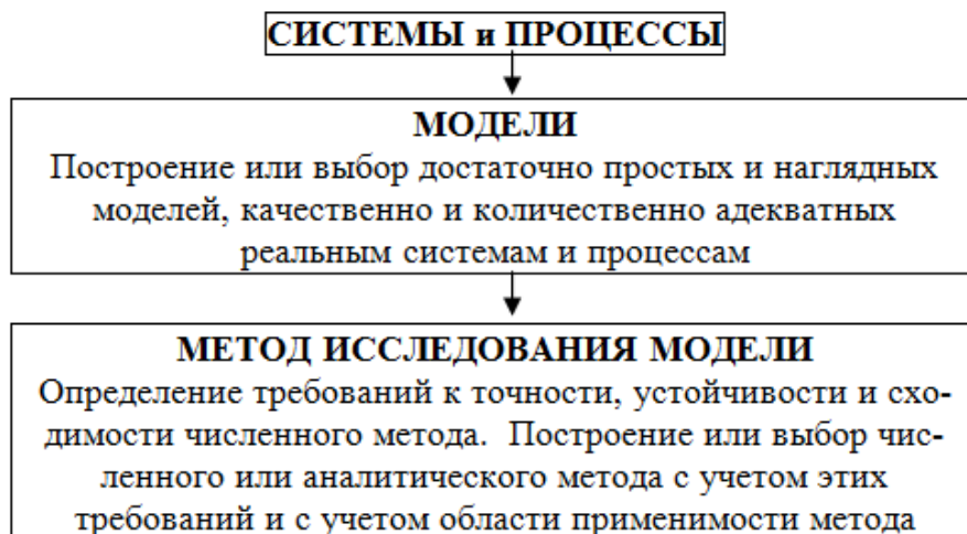
Рисунок 2 – Основные принципы моделирования
