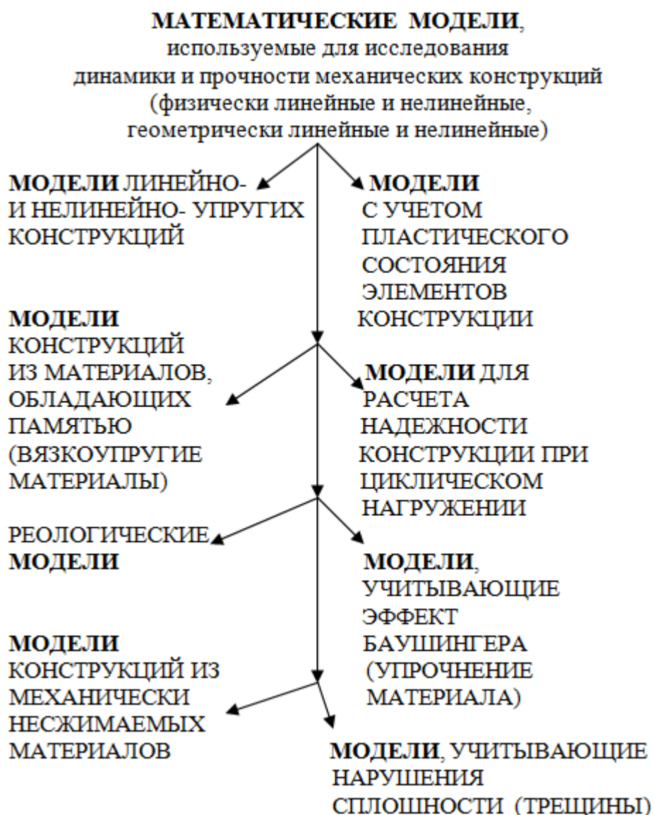
Рисунок 3 – Примеры классических моделей механики АТ и СТО
